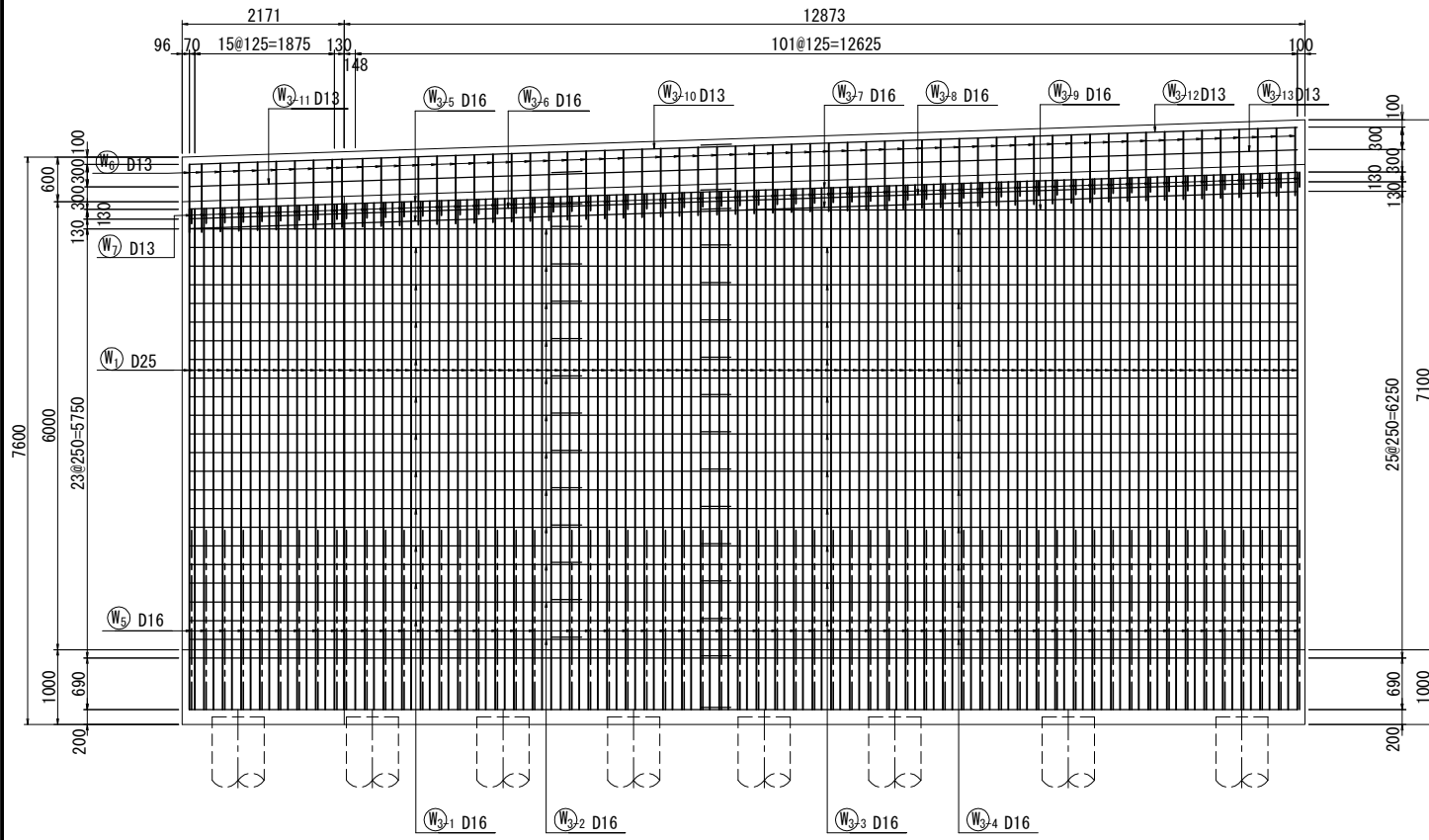
豎壁背面 (2-2)
