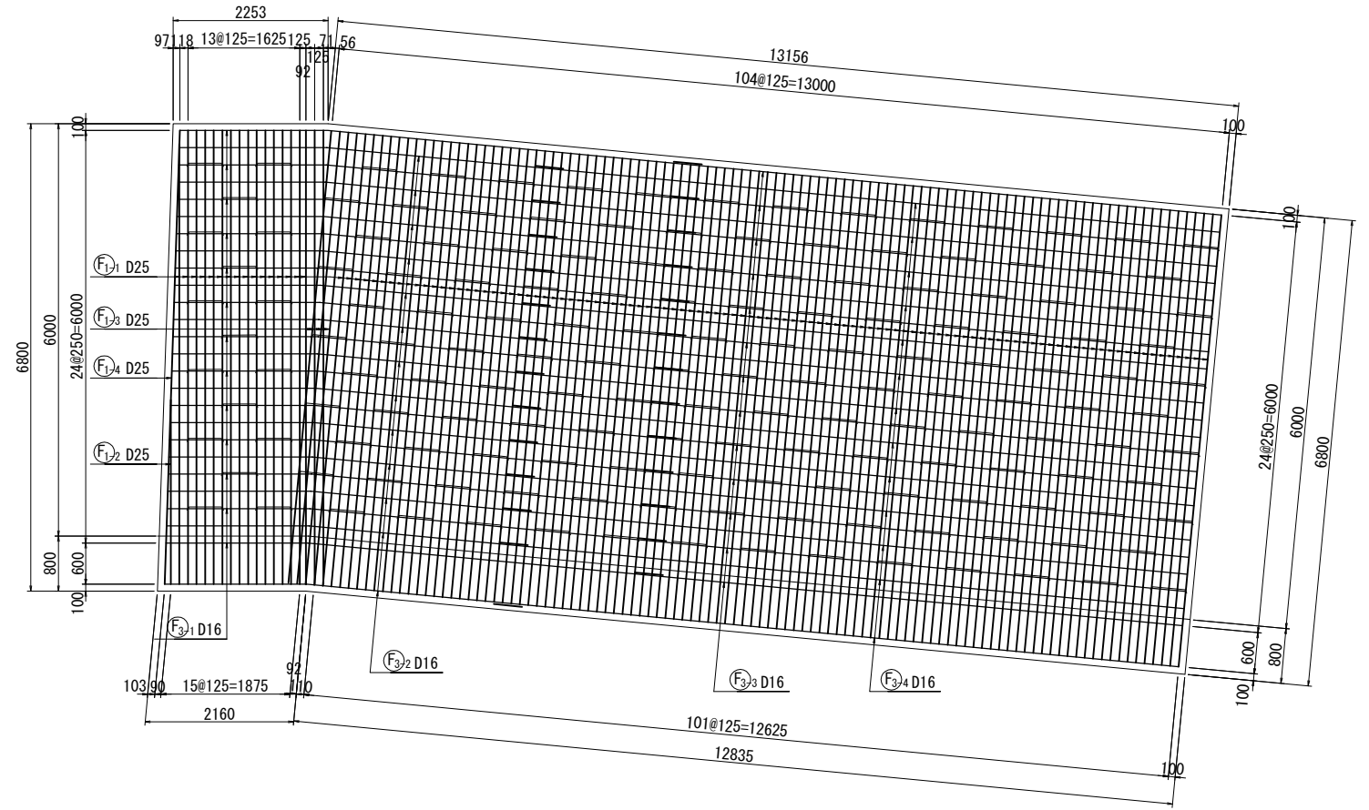
底板 (上面)
