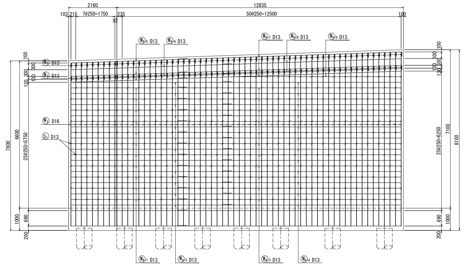
豎壁前面 (1-1)
