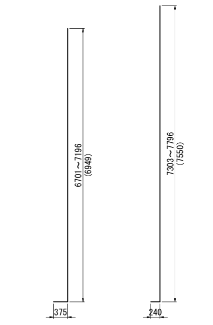
W1 120-D25x7330 (平均長) W2 61-D16x7790 (平均長)
