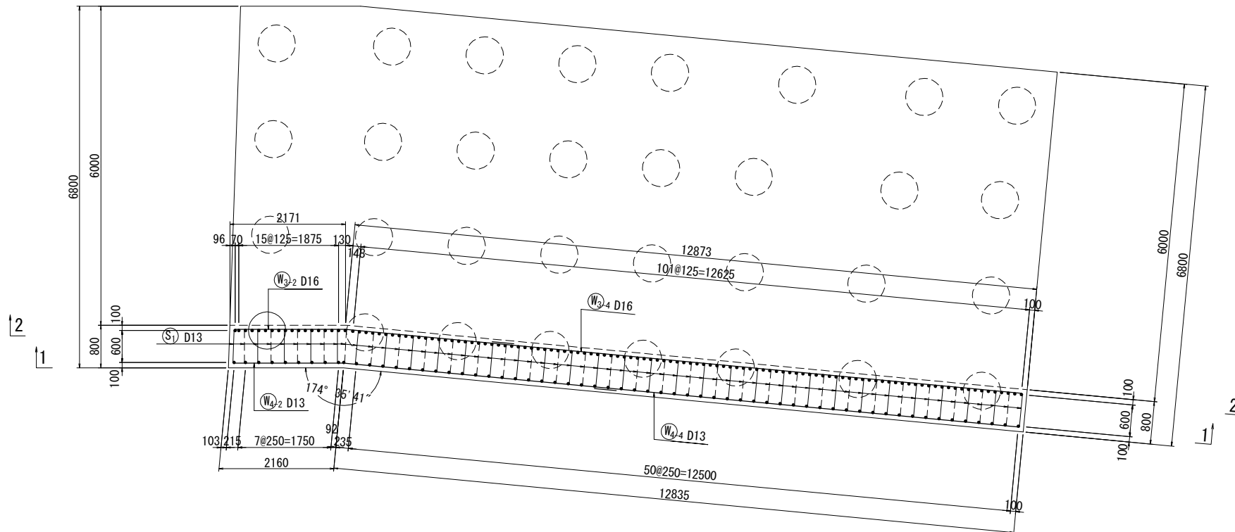
平断面図
