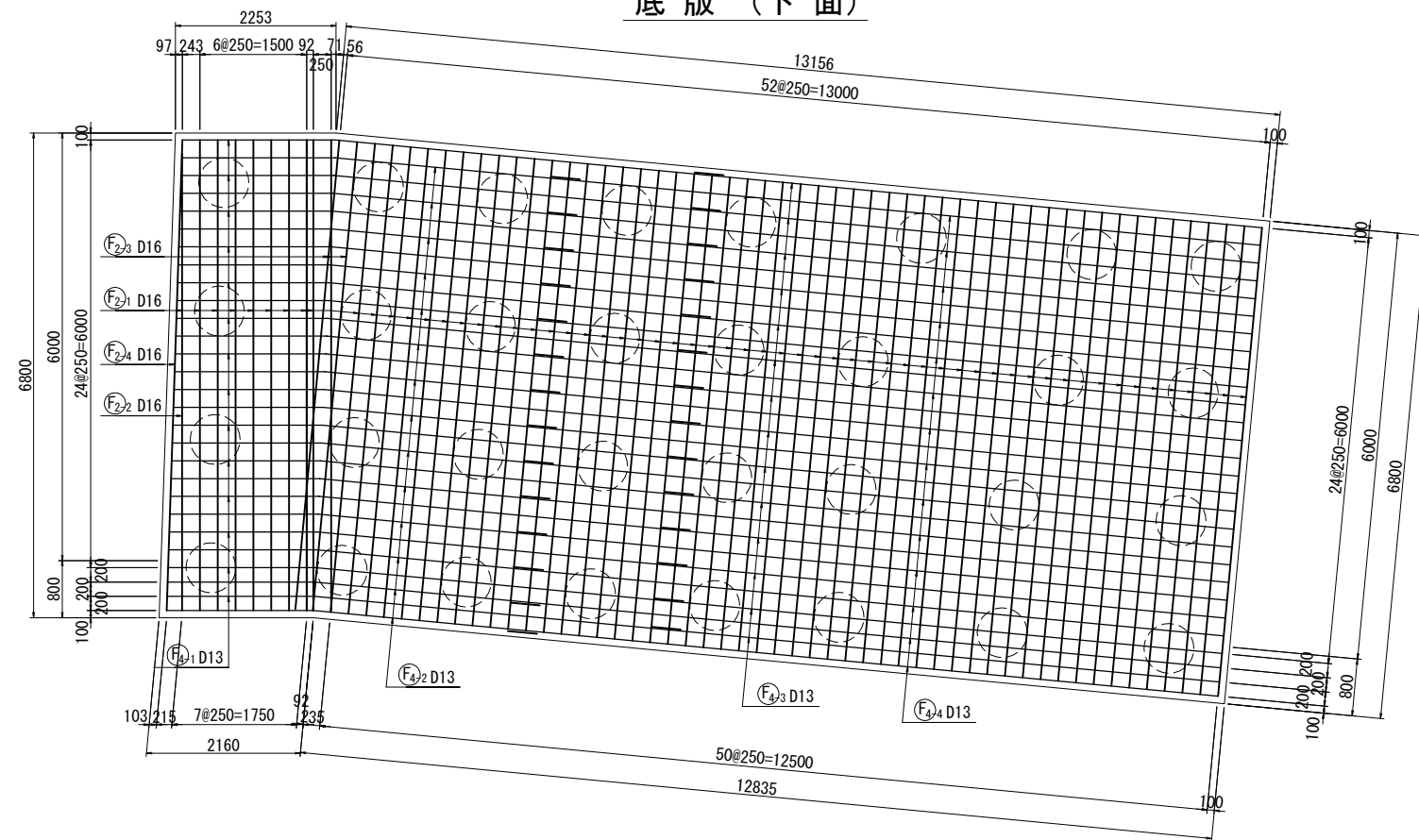
底板 (下面)
