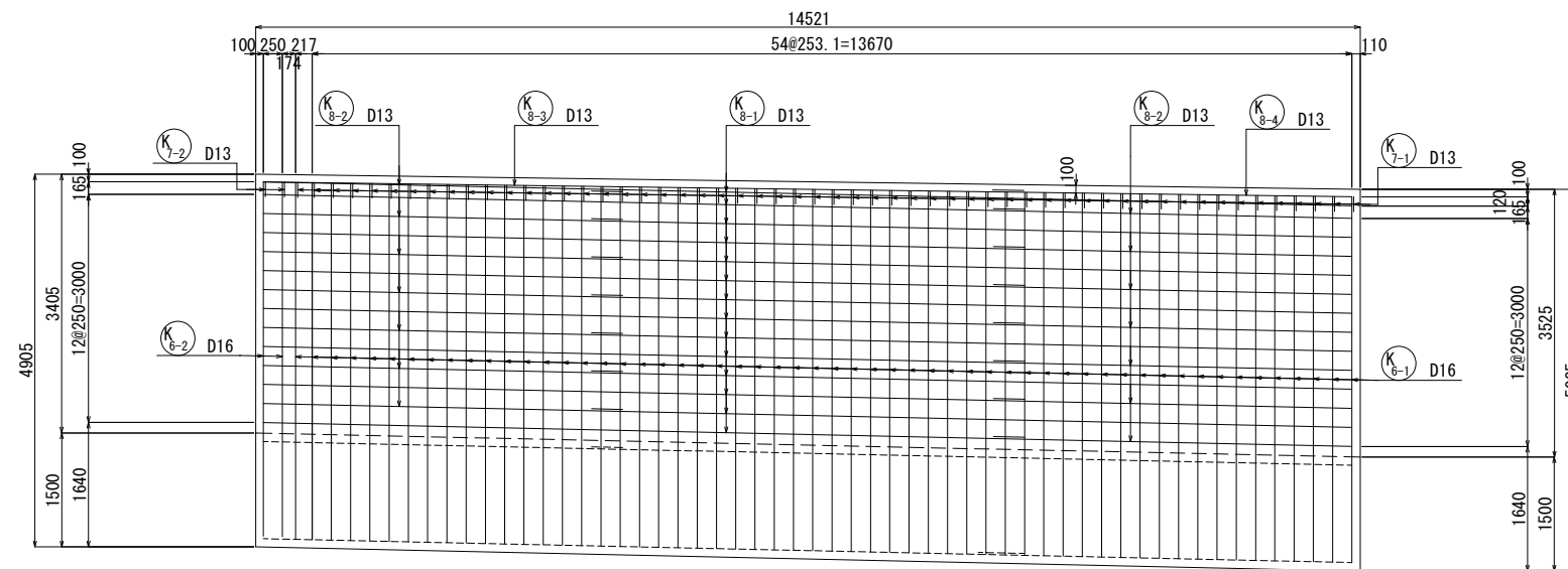
右側水路壁外面 (車道側) 6 - 6
