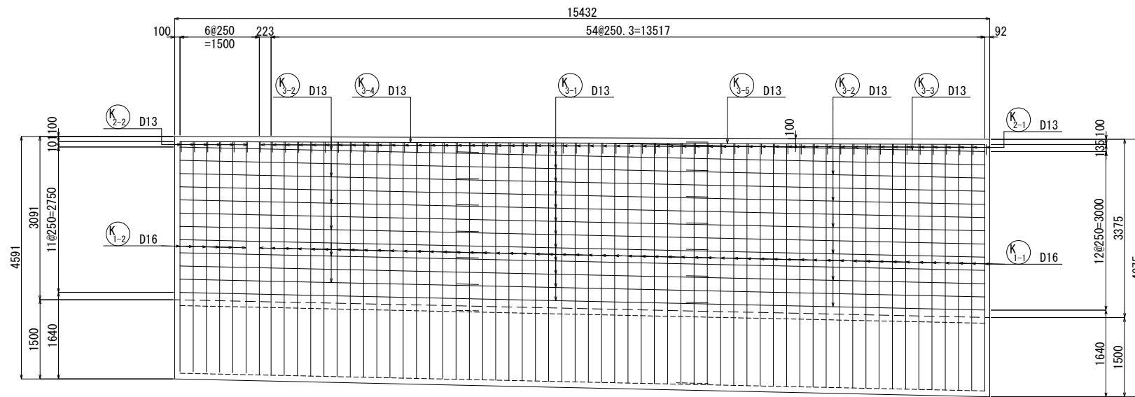
左側水路壁外面 (車道側) 4 - 4
