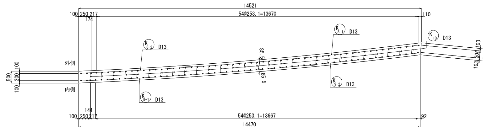
右側水路壁 F - F
