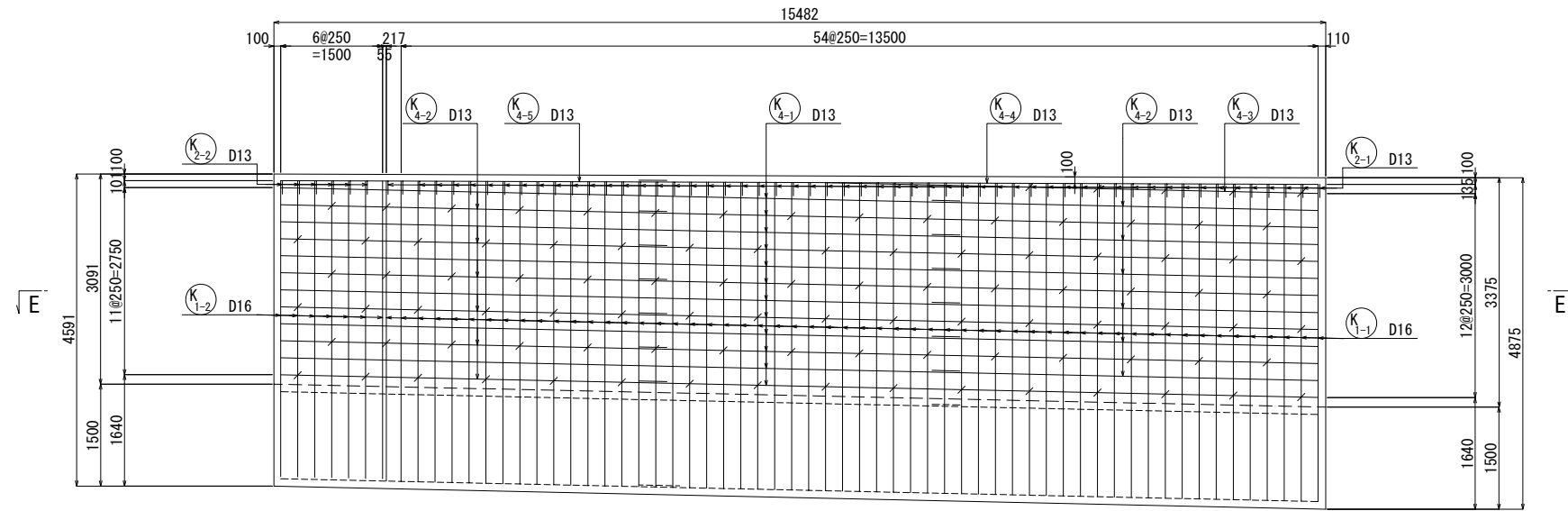
左側水路壁内面 (歩道側) 3 - 3
