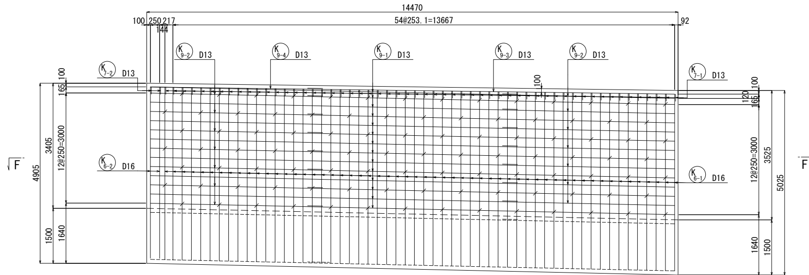
右側水路壁外面 (車道側) 6 - 6
