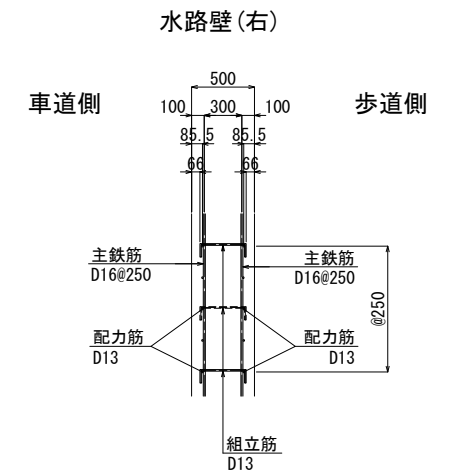
かぶり詳細図 S=1:30
