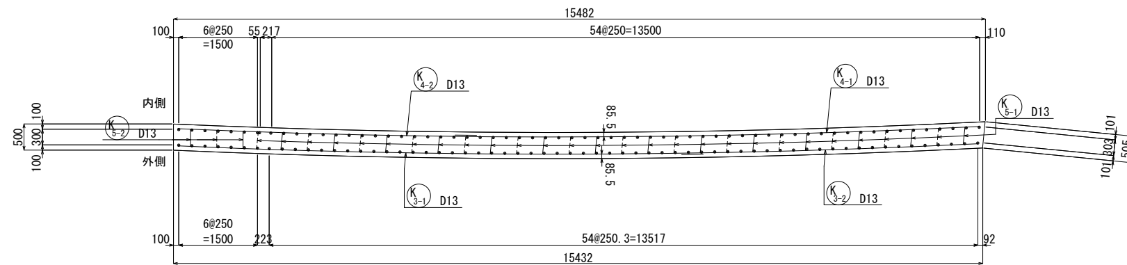
左側水路壁 E - E
